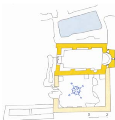
Tlocrt crkve Sv. Srđa
